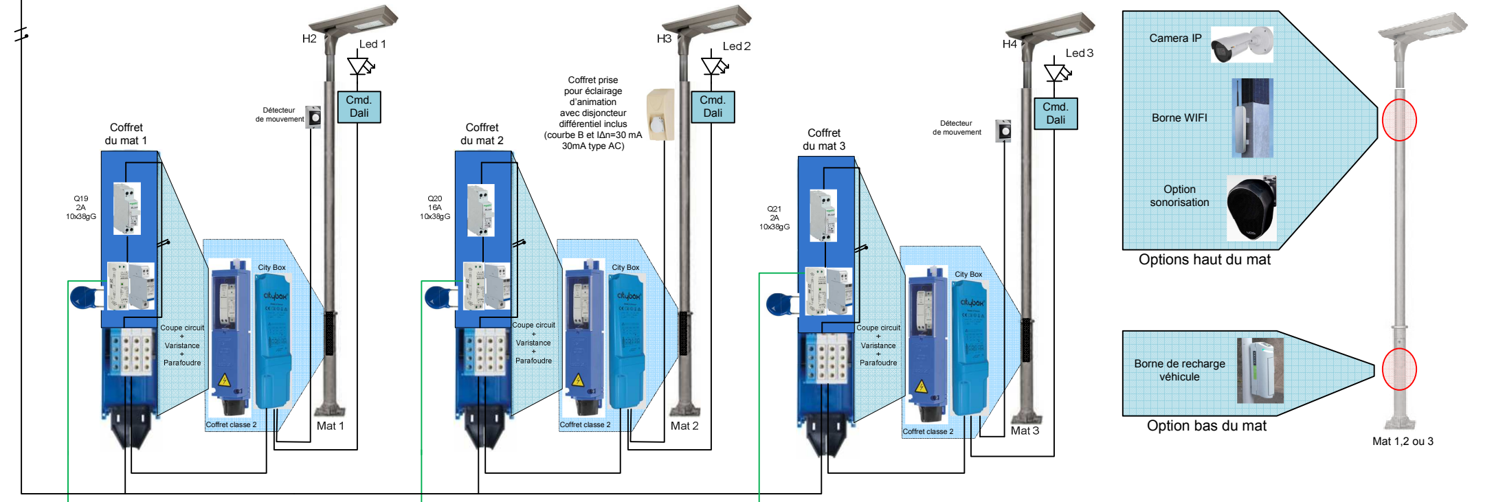
Synoptique Eclairage Type Rue
